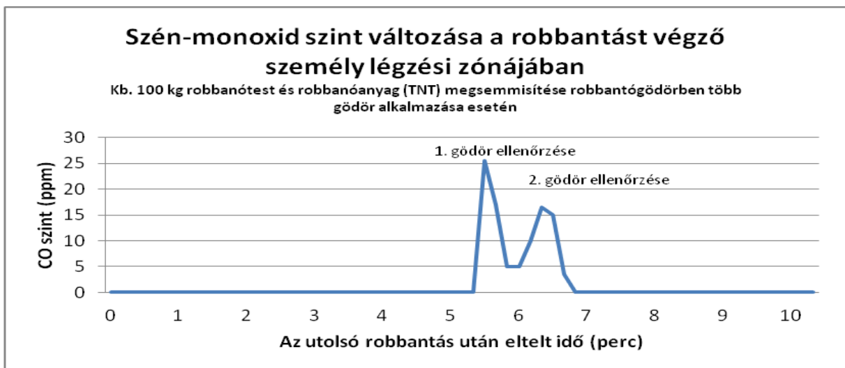
6. ábra Fel nem robbant lőszer, gránátok megsemmisítése közben mért CO-szint több robbantógödör alkalmazása esetén
