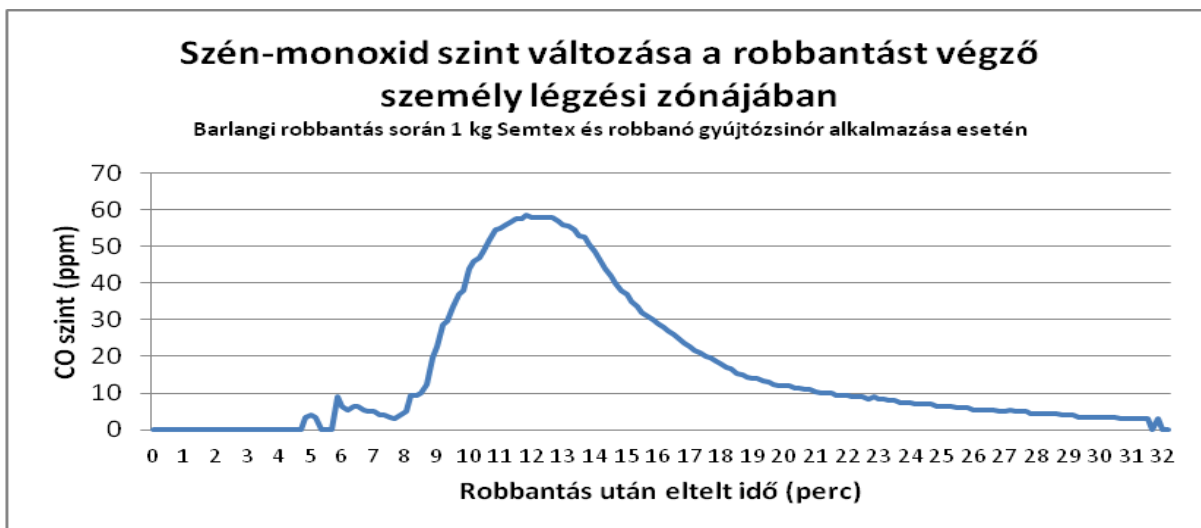
7. ábra Barlangi robbantás során 1 kg Semtexet és robbanó gyújtószinórt használtak fel
